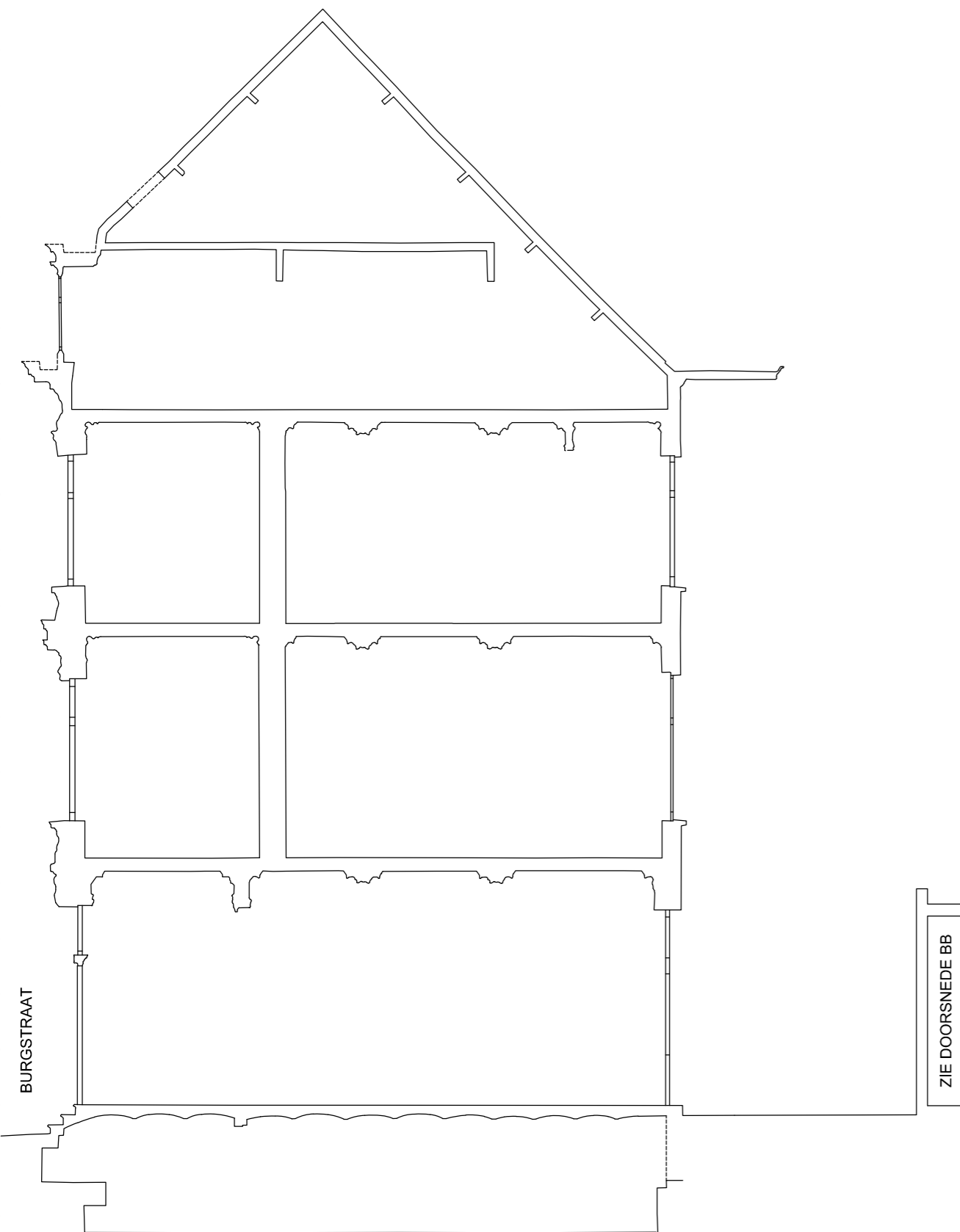
DOORSNEDE AA
