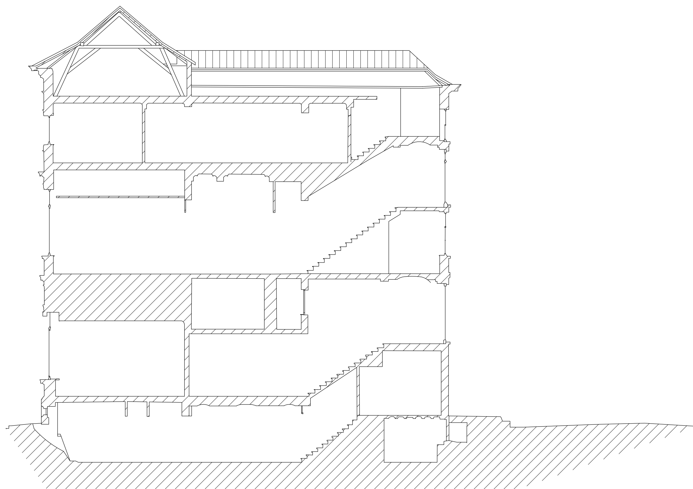
Snede 2
