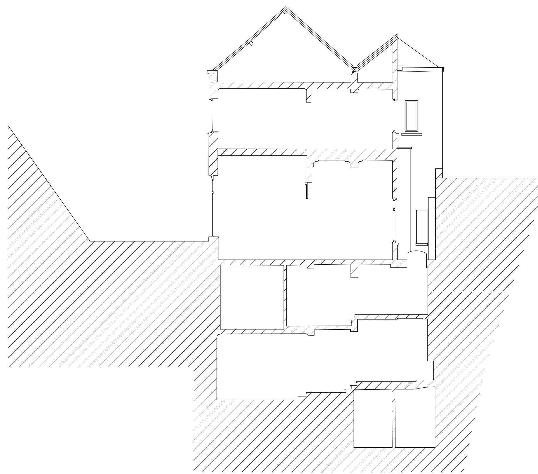
Snede 3
