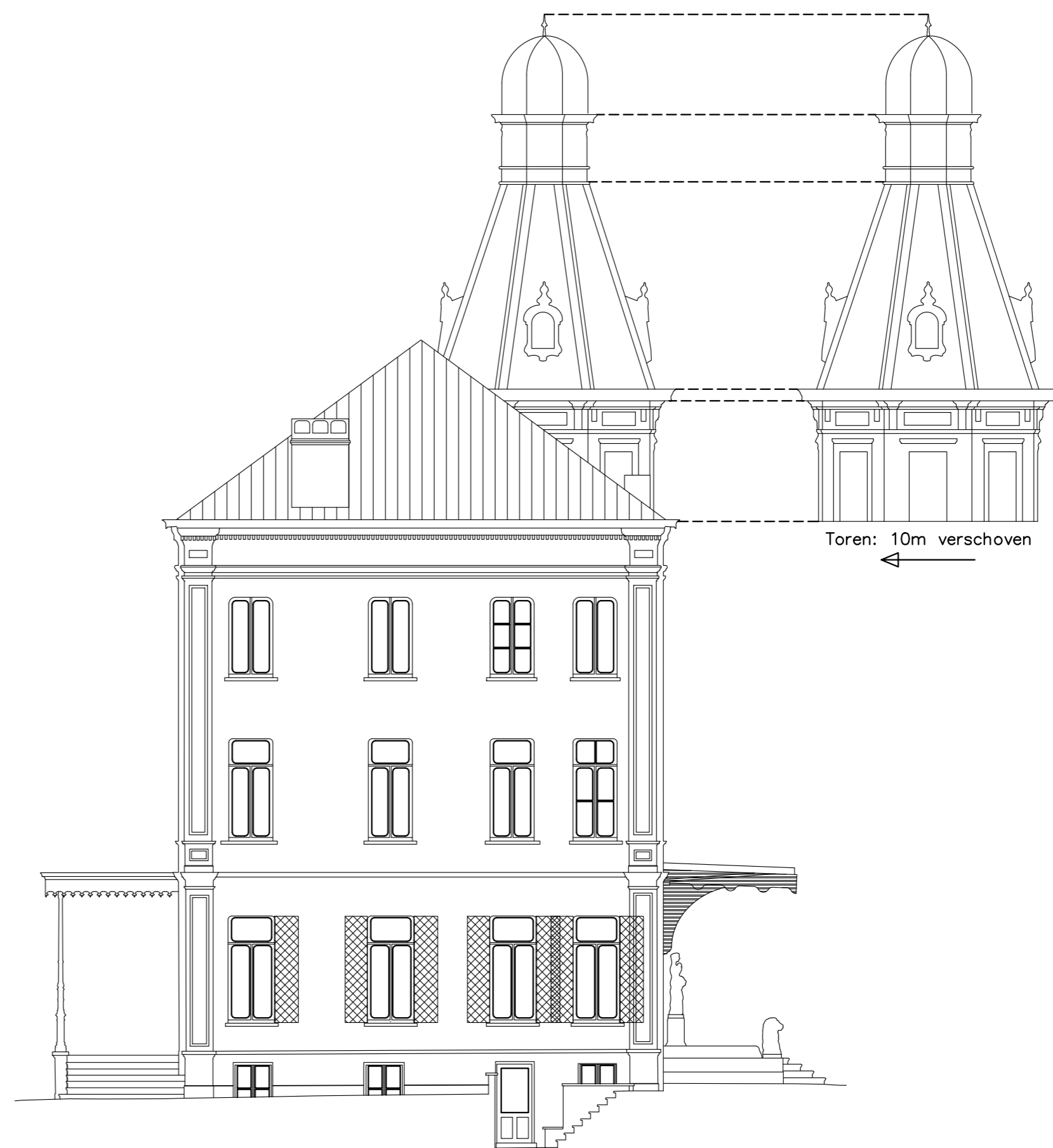
ZIJGEVEL LINKS
